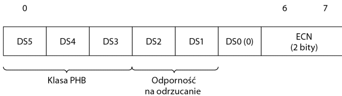
Rysunek 5.5. Znaczenie poszczególnych grup bitów DSCP, wynikające z (częściowej) kompatybilności ze znaczeniem pola Typ usługi/Klasa ruchu . W grupie standardowych DSCP bit DS0 ma zawsze wartość 0. 2-bitowe pole ECN zawiera powiadomienie dla odbiorcy, że przetworzenie datagramu odbyło się w warunkach permanentnego przeciążenia routera, co dla tegoż odbiorcy stanowić może sygnał dla podjęcia stosownych działań, np. zażądania od nadawcy spowolnienia tempa transmisji
